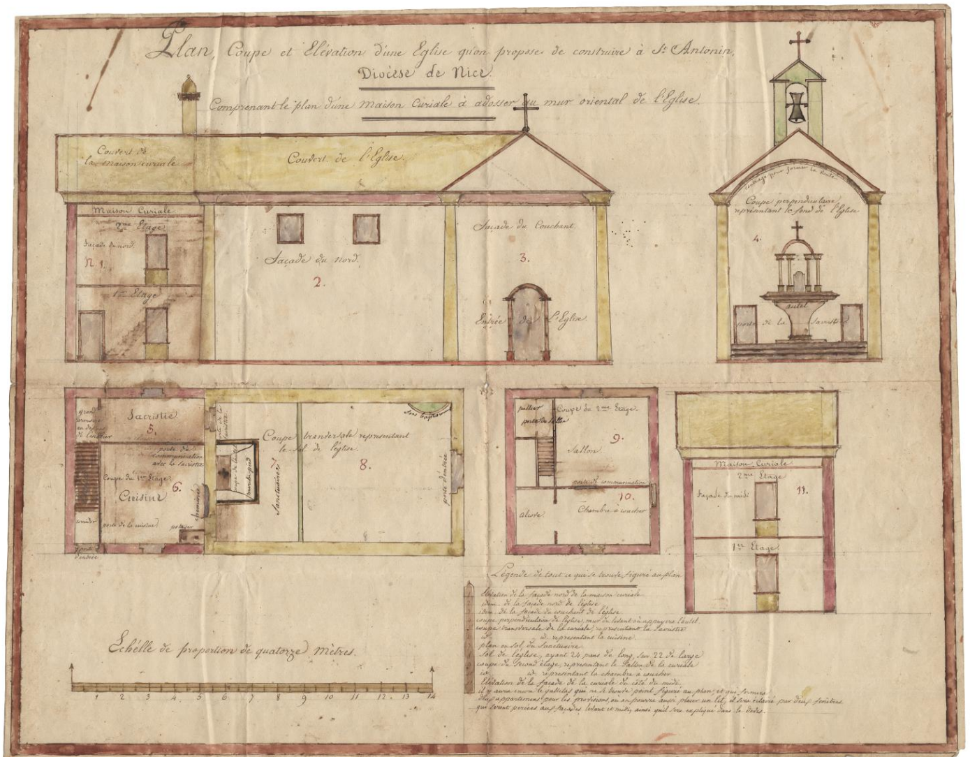
Figure 12. Plan, coupe et élévation pour l'église de Saint-Antonin, 1 FS 1258
