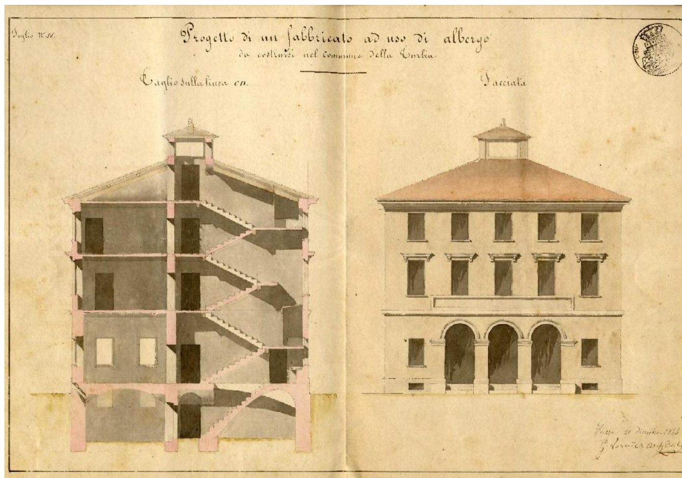
Figure 13. Figure 14. Plan pour la construction d'un hôtel à La Turbie, 1 FS 1314
