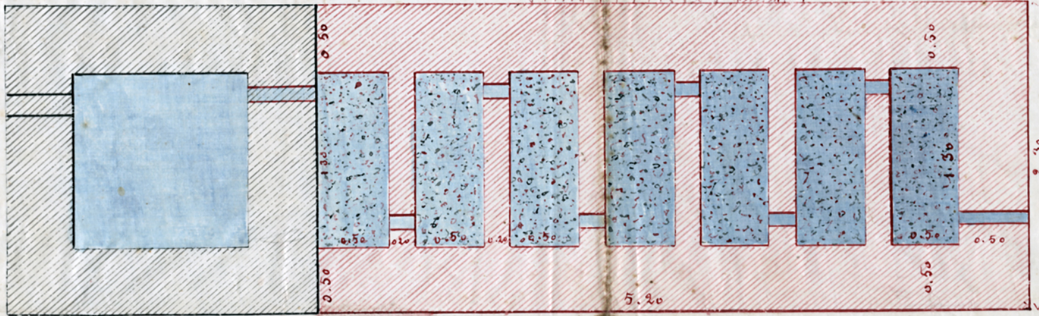
Plan de la Chambre de captage.
