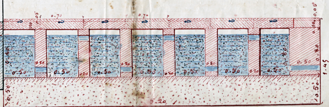
Coupe en long du Filtre.
