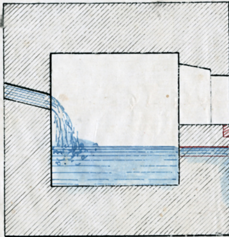
Coupe en travers de la chambre de captage des eaux.
