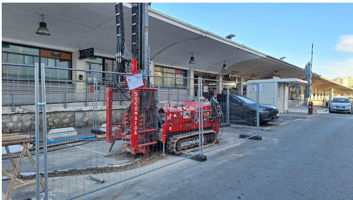
Travaux de sondages géotechniques, Marseille Saint Charles
